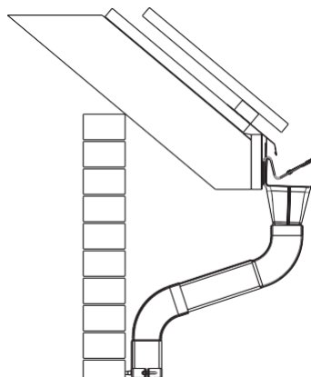
ПОПЕРЕЧНИЙ РОЗРІЗ МОНТАЖУ ДАХУ З КАРНИЗЕМ
