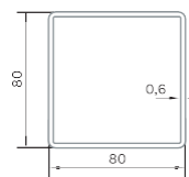
РОЗРІЗ ТРУБИ
