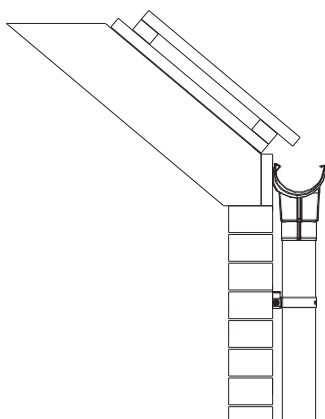
ПОПЕРЕЧНИЙ МОНТАЖ РОЗРІЗУ ДАХУ БЕЗ КАРНИЗУ
