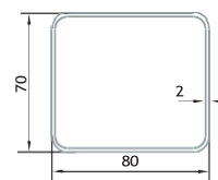
РОЗРІЗ ТРУБИ
