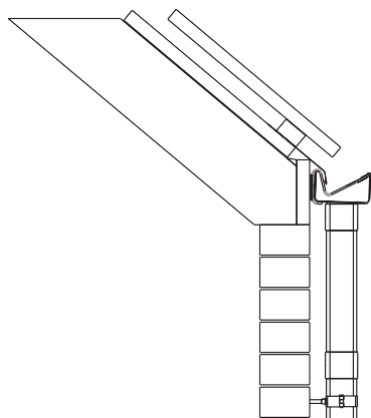
ПОПЕРЕЧНИЙ РОЗРІЗ МОНТАЖУ ДАХУ БЕЗ КАРНИЗУ
