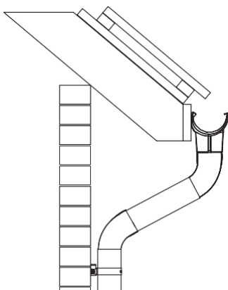
ПОПЕРЕЧНИЙ МОНТАЖ РОЗРІЗУ ДАХУ З КАРНИЗЕМ
