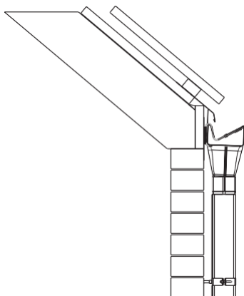
ПОПЕРЕЧНИЙ РОЗРІЗ МОНТАЖУ ДАХУ БЕЗ КАРНИЗУ
