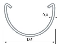
РОЗРІЗ РИНВИ
