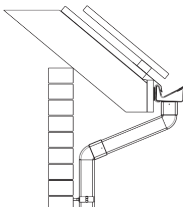
ПОПЕРЕЧНИЙ РОЗРІЗ МОНТАЖУ ДАХУ З КАРНИЗЕМ
