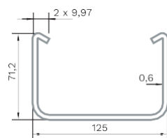
РОЗРІЗ РИНВИ
