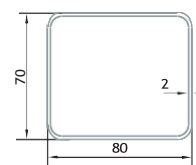
РОЗРІЗ ТРУБИ
