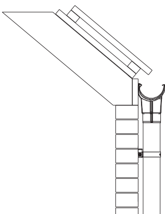
ПОПЕРЕЧНИЙ МОНТАЖ РОЗРІЗУ ДАХУ БЕЗ КАРНИЗУ
