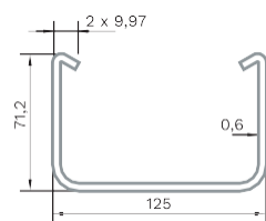
РОЗРІЗ РИНВИ
